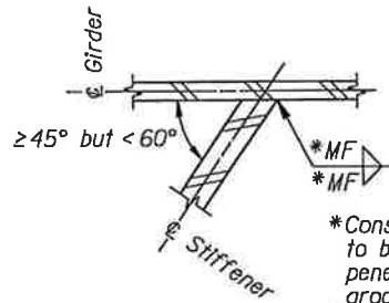
CASE III (Bevel Stiffener)
