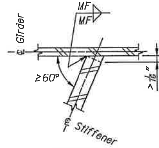
CASE II (Bevel Stiffener)
