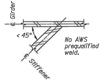
CASE IV (Bevel Stiffener)
